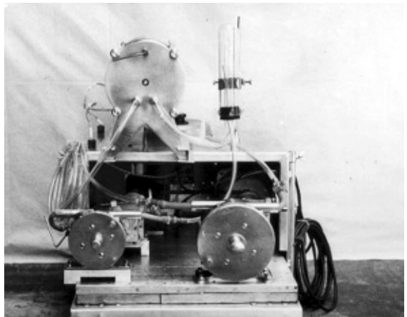
Máquina de circulação extracorpórea, com bomba de rolete e oxigenador de discos tipo Kay-Cross, utilizada na primeira cirurgia com circulação extracorpórea total.
